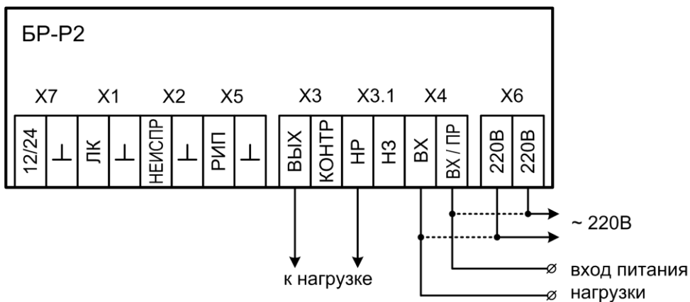
Рис.В7 Универсальная замыкающая схема подключения. Питание БР-Р2 от сети 220 В. Пунктиром показан вариант питания нагрузки от входа 220В БР-Р2
