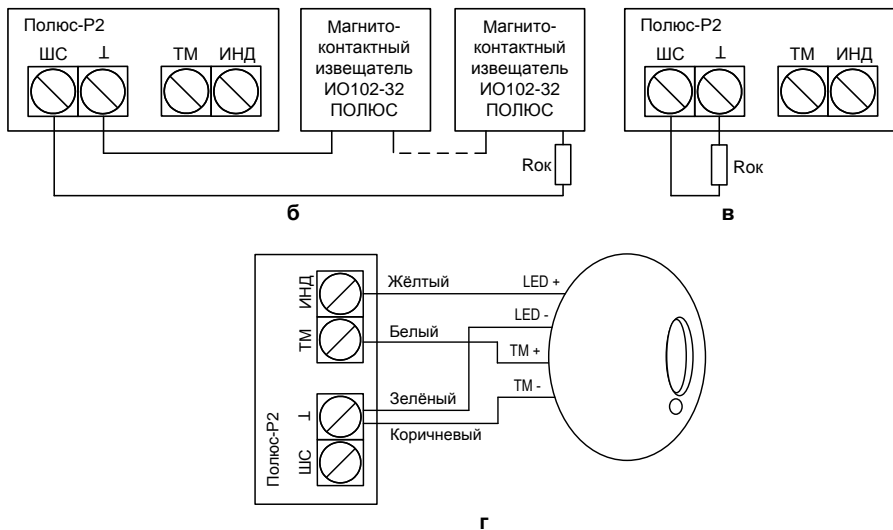
Рис.11б, в, г Схемы подключений к ПОЛЮС-Р2
