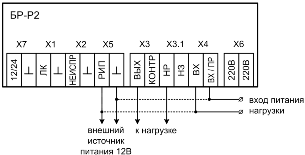
Рис.В6 Универсальная замыкающая схема подключения. Питание БР-Р2 от РИП 12 В. Пунктиром показан вариант питания нагрузки от входа РИП БР-Р2
