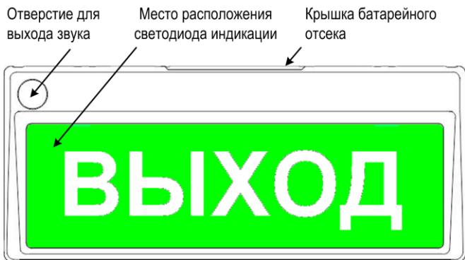
Рис.3.16 Оповещатель Призма-P2M вариант 2. Внешний вид
