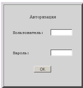
Рисунок 12.5 – Окно авторизации
