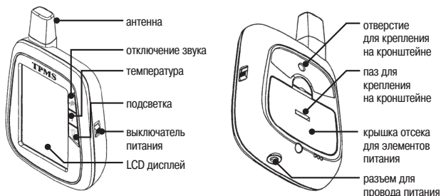
Расположение элементов управления и внешний вид приёмного устройства
