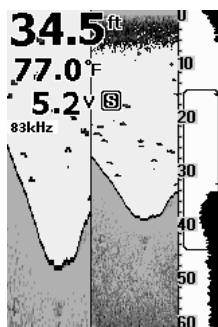
ЭКРАН ЭХОЛОТА С МАСШТАБИРОВАНИЕМ (83 КГц)
