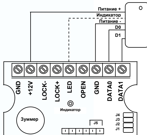
Пример подключения считывателя RFID по Wiegand 26
