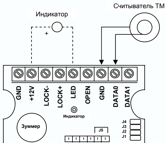
Пример подключения считывателя TM
