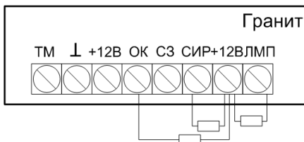
Рисунок 2.2 – Установка оконечных резисторов 7,5 кОм
