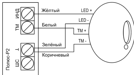
Рисунок 3.5 – Подключение порта ТМ
