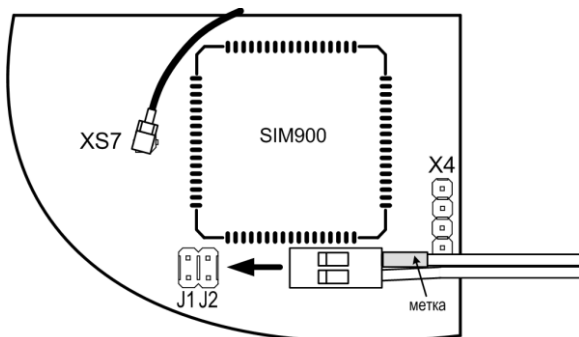
Рисунок 3.8 – Подключение термодатчика
