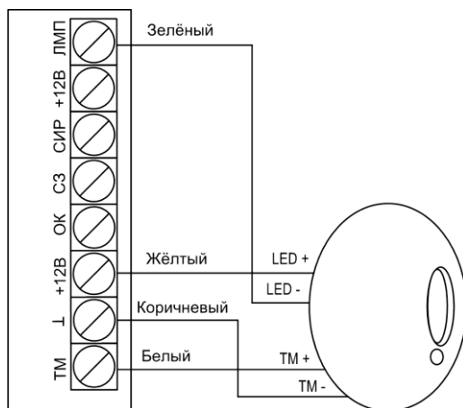
Рисунок 2.1 – Подключение порта ТМ к прибору
