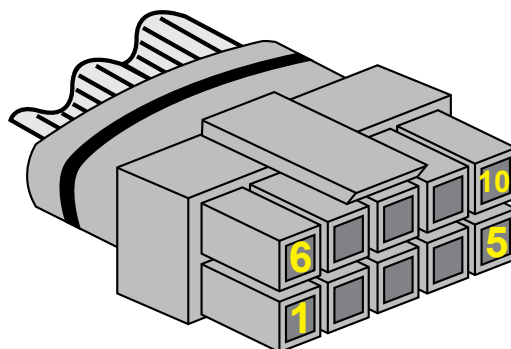
Рис. 2.1. Разъем 10-контактного интерфейсного кабеля
