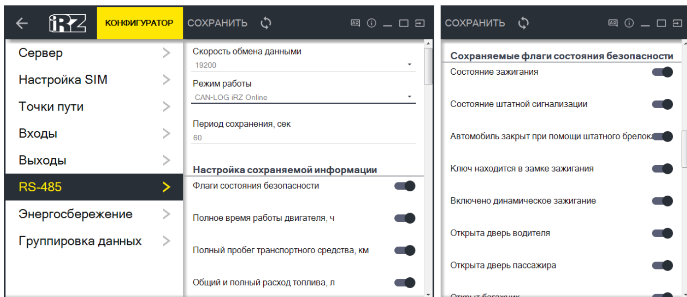
Рис. 4.9. Вкладка «RS-485» (режим «CAN-LOG iRZ Online»)
