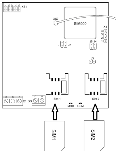
Рисунок 3.13 – Коммуникатор
