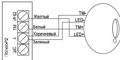
Рисунок 3.6 – Подключение порта ТМ
