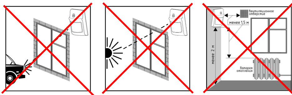
Рисунок 3.4 – Схемы неверного расположения устройства
