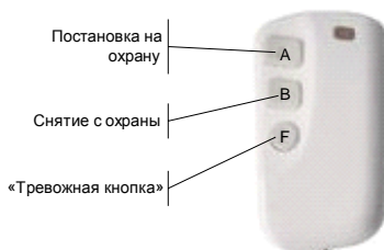
Рисунок 3.1 – Брелок БН-Р2
