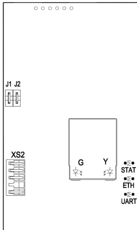
Рисунок 3.15 – IP регистратор
