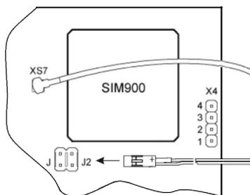
Рисунок 3.14 – Подключение термодатчика
